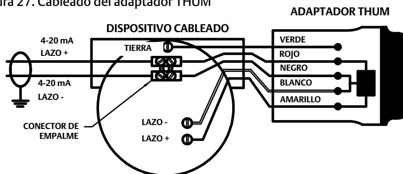
Figura 27. Cableado del adaptador THUM
