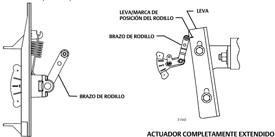
Figura 6. Variación del brazo de rodillo utilizado para actuadores de vástago deslizante (lineales) con una carrera superior a 210 mm (8.25 in.)
