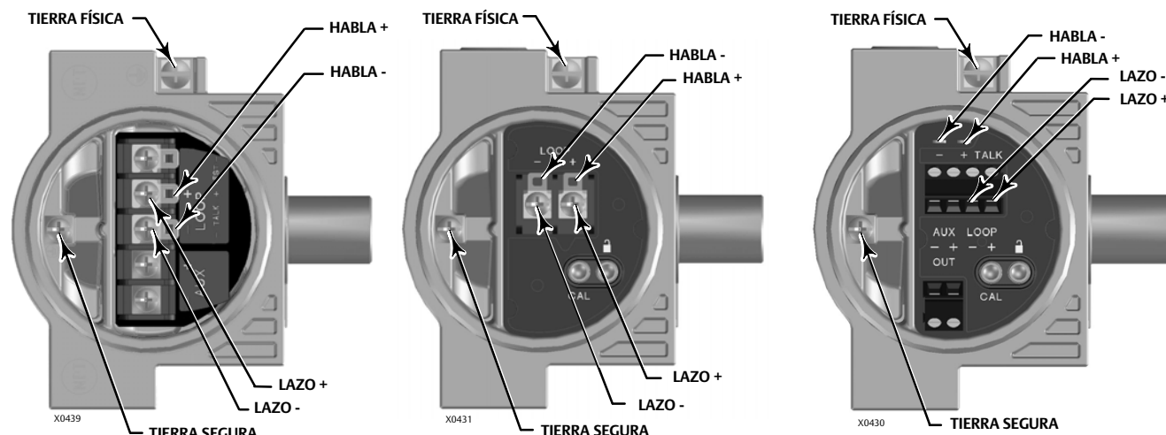
Figura 21. Conexiones de lazo y de habla
