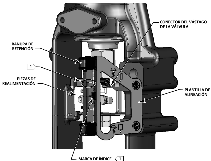
Figura 7. Alineación del conjunto del imán de aire para abrir
