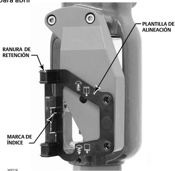
Figura 3. Alineación del conjunto del imán de aire para abrir
