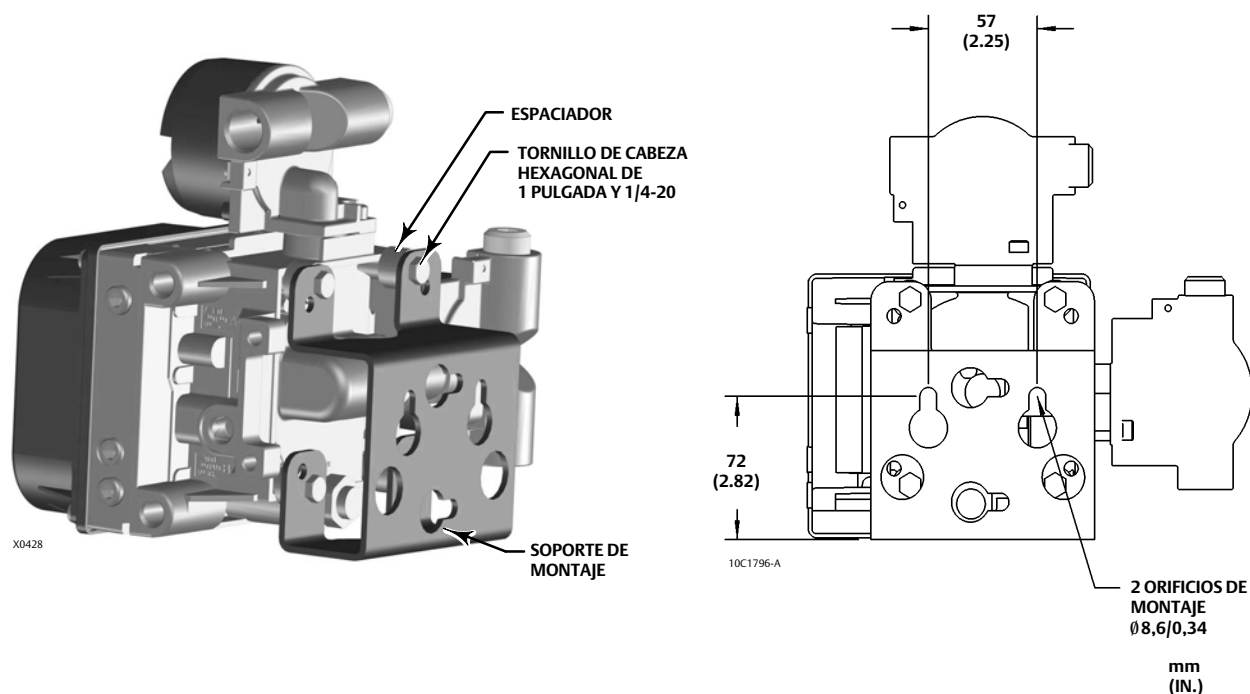
Figura 15. Montaje en pared del FIELDVUE DVC6205
