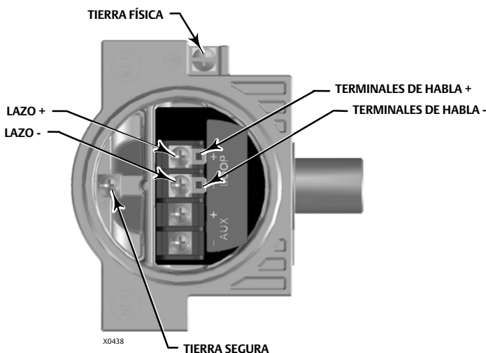
Figura 19. Caja de terminales de conexiones del lazo
