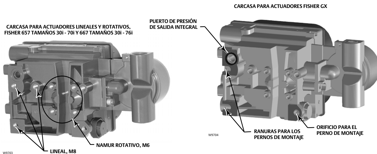
Figura 1. Variaciones de carcasa
