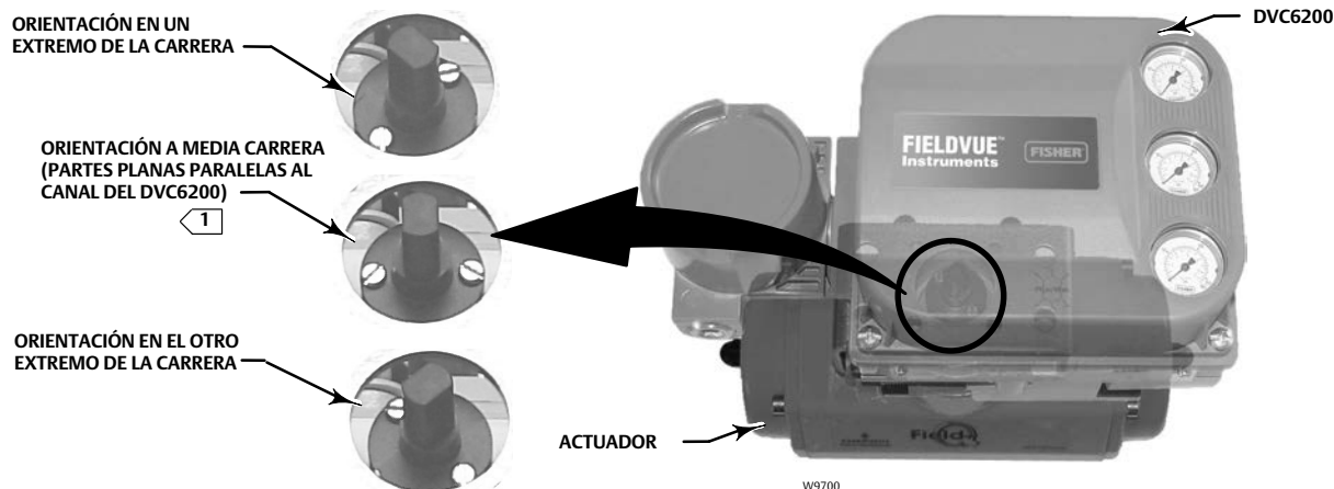
Figura 13. Orientación del conjunto del imán en los actuadores de cuarto de vuelta
