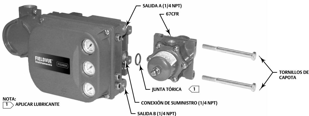
Figura 16. Montaje integral de un regulador Fisher 67CFR en un controlador de válvula digital FIELDVUE DVC6200
