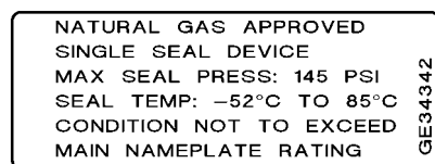
Figura 18. Etiqueta de la caja de terminales certificada para gas natural
