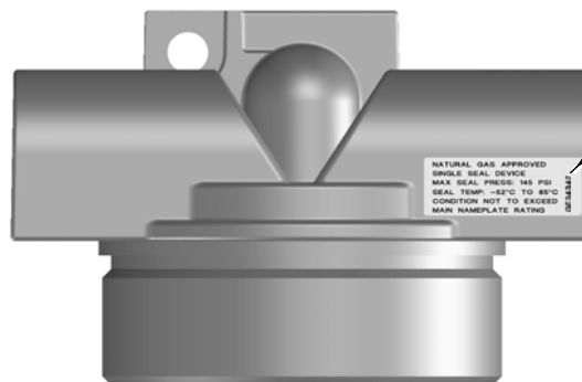
Figura 18. Etiqueta de la caja de terminales certificada para gas natural
