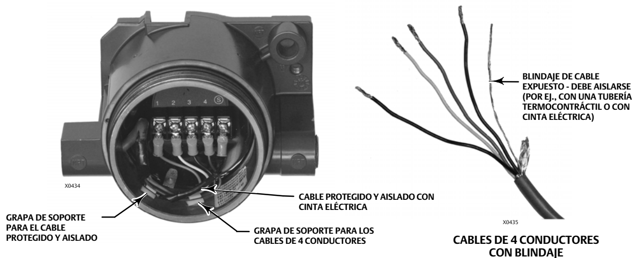
Figura 25. Grapas de cables
