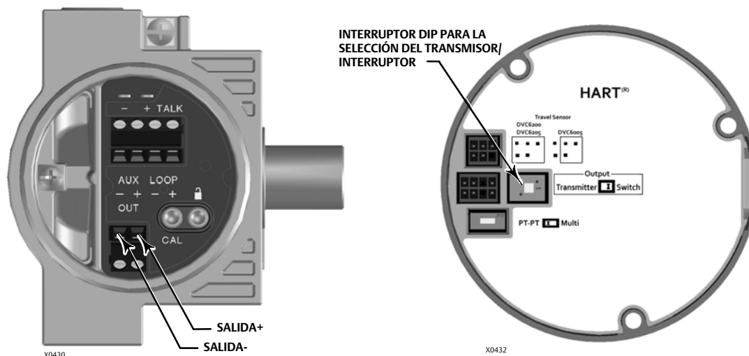
Figura 22. Conexiones de SALIDA y configuración del transmisor/interruptor
