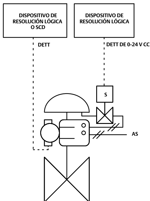
Figura 32. Controlador de válvula digital y válvula solenoide energizados por separado
