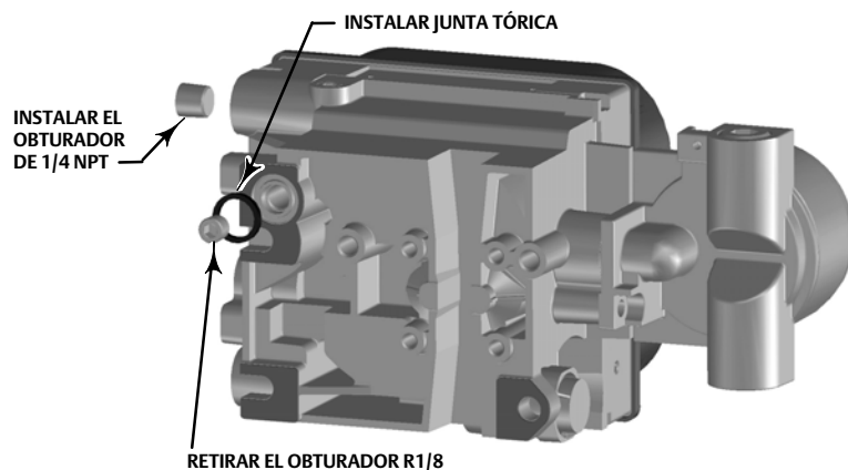
Figura 8. Modificaciones para el actuador de montaje integral; solo la construcción de aire para abrir
