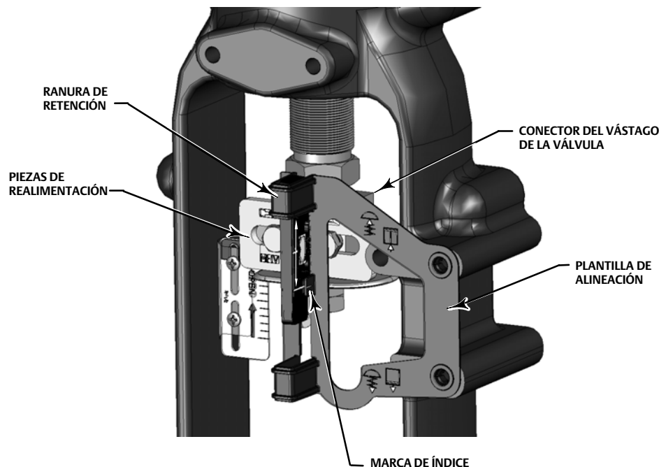
Figura 9. Alineación del conjunto del imán de aire para cerrar
