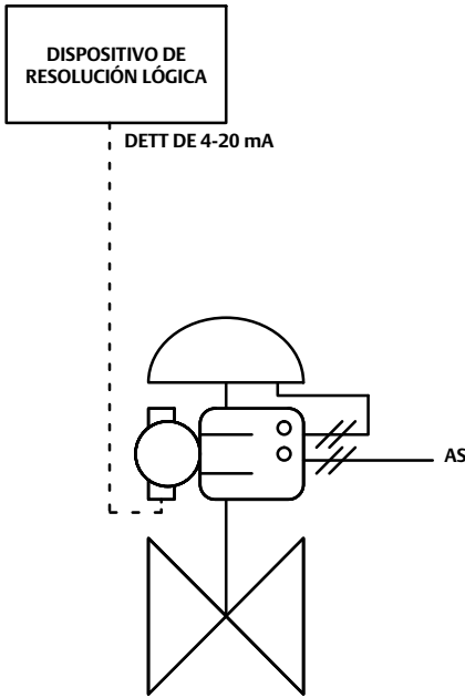
Figura 30. FIELDVUE DVC6200 SIS alimentado con 4-20 mA
