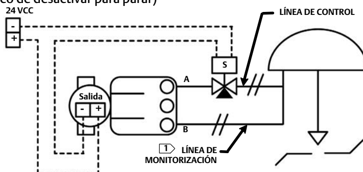
Figura 37. Conexión de la válvula de solenoide para prueba de la válvula de solenoide según el DVC6200 SIS (se muestra el circuito neumático de desactivar para parar)
