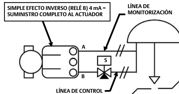
Figura 36. Tubería para monitorización de la condición operativa de la válvula solenoide, controlador de válvula digital tipo energizar para activar
