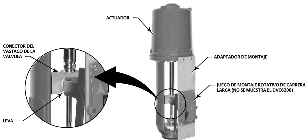
Figura 5. Montaje en actuadores de vástago deslizante (lineales) con una carrera superior a 210 mm (8.25 in.)
