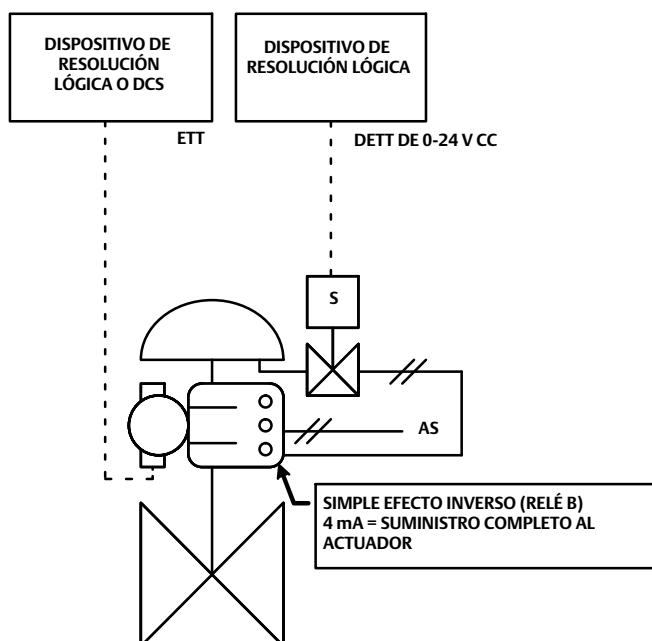
Figura 34. SIS FIELDVUE DVC6200 y válvula de solenoide alimentados por separado
