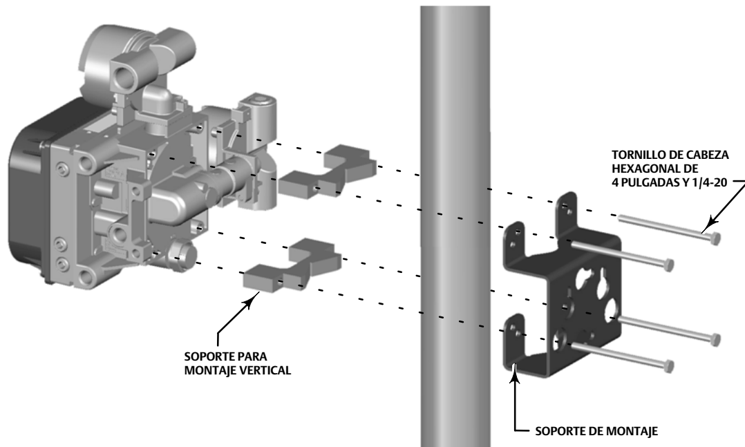
Figura 14. Montaje en el soporte de tubería del FIELDVUE DVC6205
