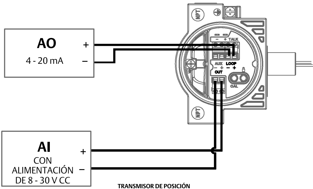
Figura 23. FIELDVUE DVC6200 con transmisor de posición o interruptor discreto, esquema de cableado en el campo
