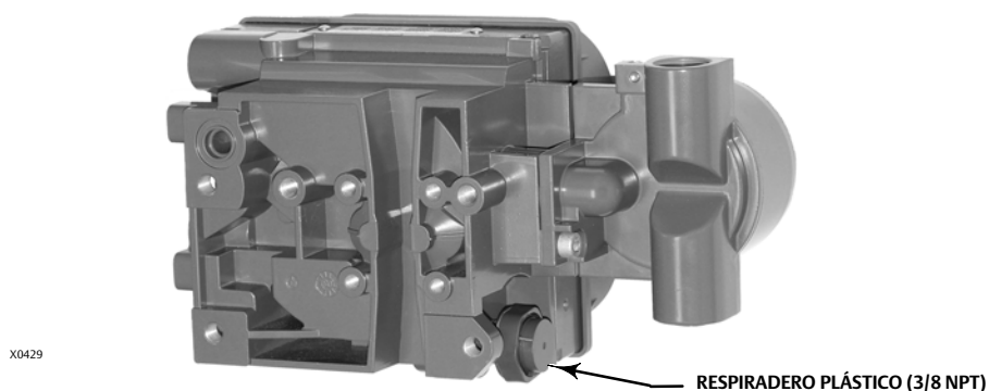
Figura 17. Conexión de ventilación
