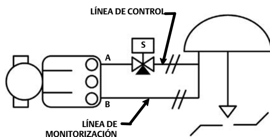
Figura 35. Tubería para monitorización de la condición operativa de la válvula de solenoide, controlador de válvula digital tipo des-energizar para activar
