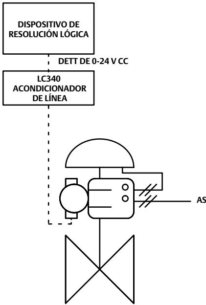
Figura 31. FIELDVUE DVC6200 SIS alimentado con 0-24 VCC
