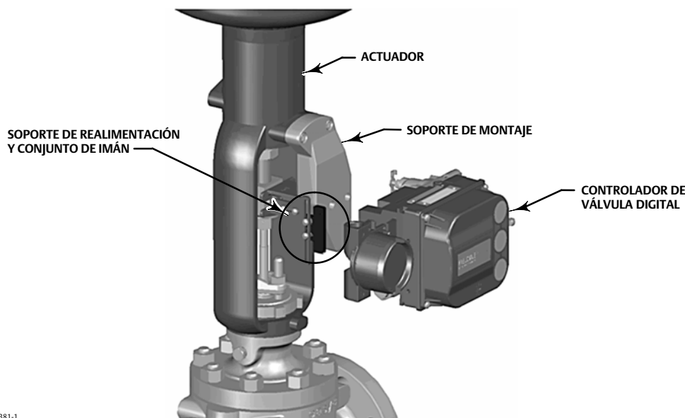
Figura 2. Piezas de montaje para actuadores de vástago deslizante con una carrera máxima de 210 mm (8.25 in.)
