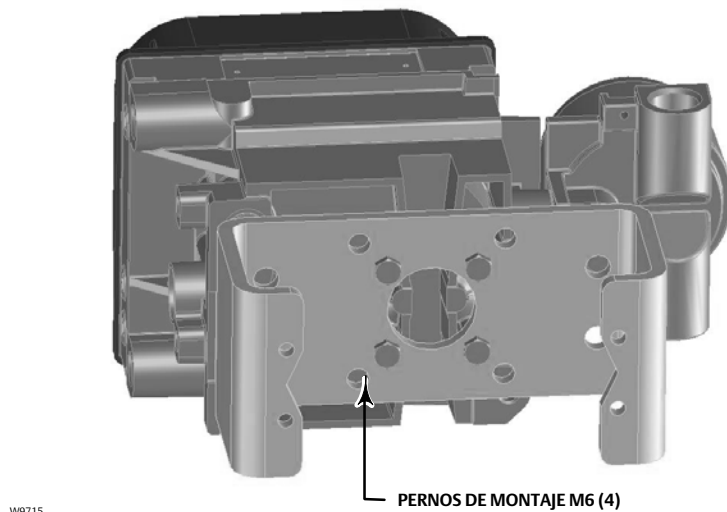
Figura 12. Montaje en actuadores de cuarto de vuelta
