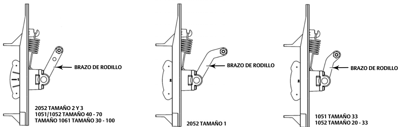
Figura 11. Variaciones de montaje de actuadores rotativos
