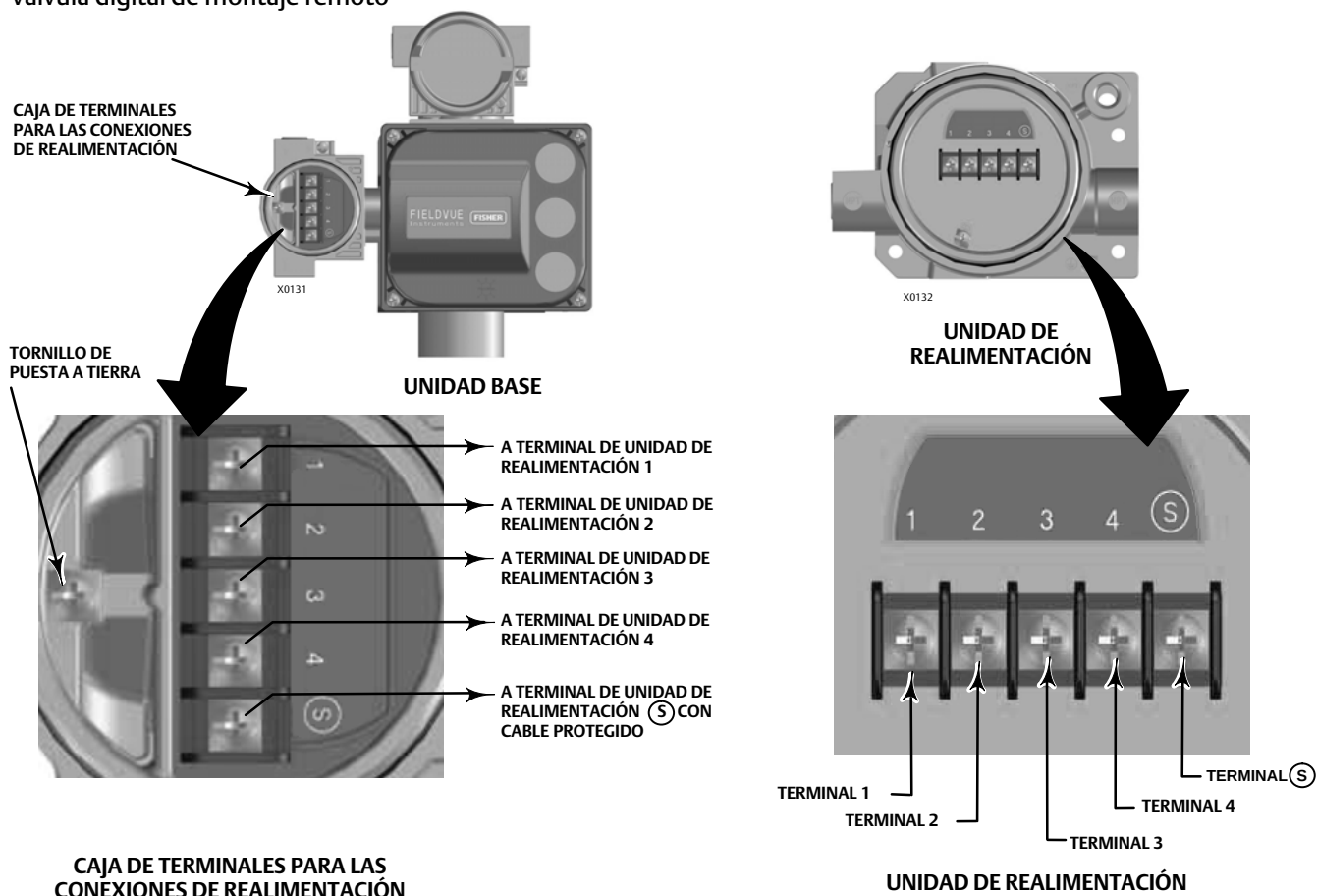
Figura 24. Detalles de terminales para conectar la unidad base y la unidad de realimentación en controladores de válvula digital de montaje remoto
