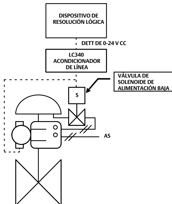
Figura 33. SIS FIELDVUE DVC6200 y válvula de solenoide alimentados de forma conjunta
