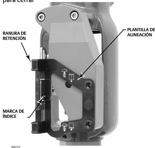
Figura 4. Alineación del conjunto del imán de aire para cerrar
